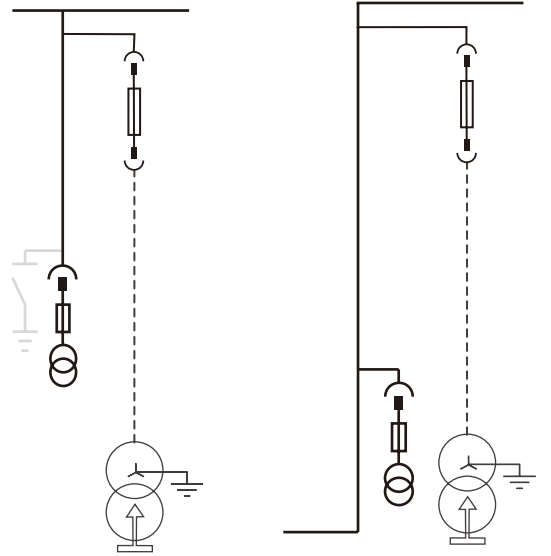
1 M-带接地变压器的PT单元
