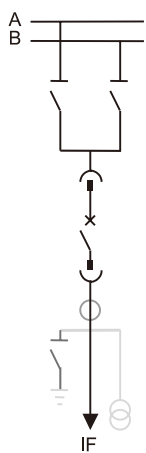
1 IF-进线/馈线单元
