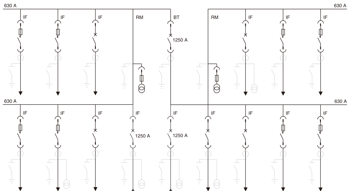
纯双层柜组合方案
