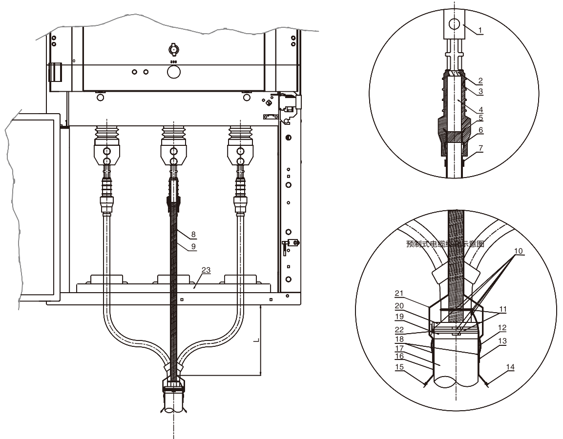
图17.5: 电缆连接示意图
