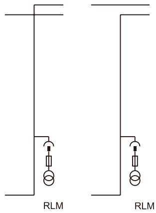
8 RLM-带 PT 手车纵向提升单元
