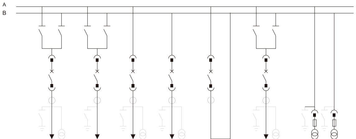
带母联开关的双母线系统
