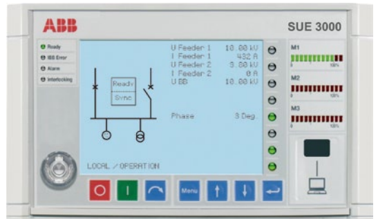
快速切换系统：3台断路器的配置，带母联。当缺少任何一路的电能供应，母联断路器合闸和失电的进线断路器的分闸命令同时发出。
