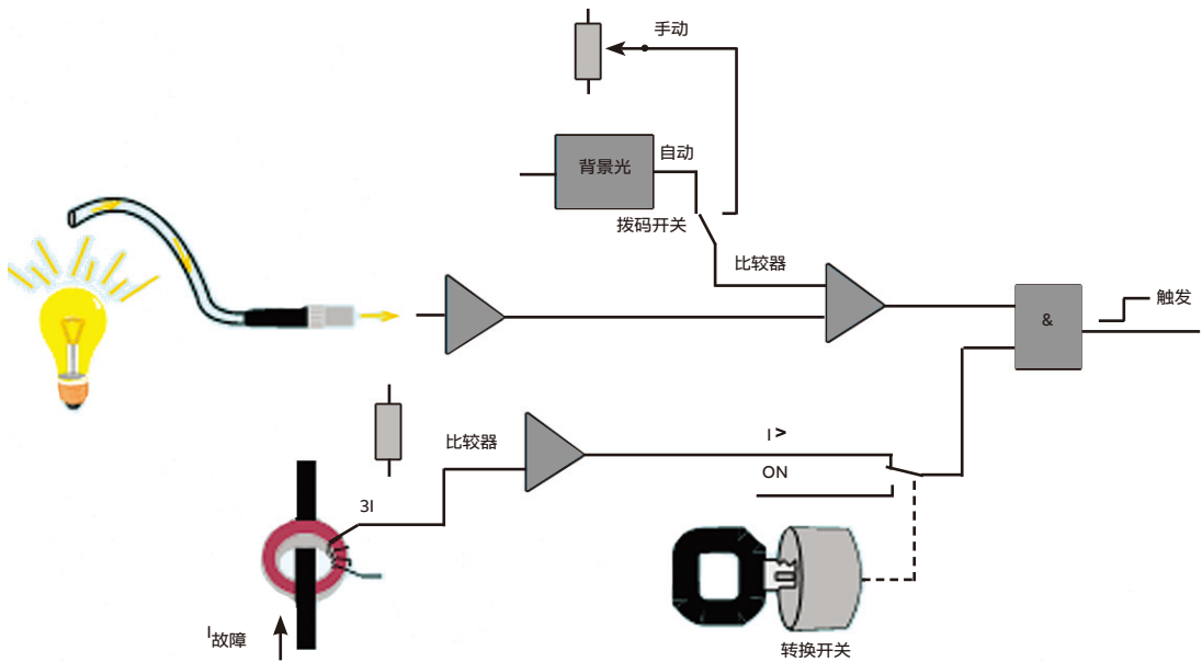
— 判据逻辑示意图
