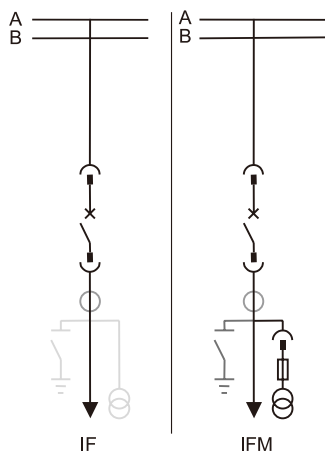
2 IF/IFM-母线A进线(复式)
