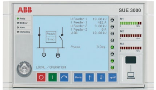
快速切换系统：两台断路器的配置，无母联。如果工作进线失去电源供应，工作进线分闸和备用进线合闸的命令同时发出。
