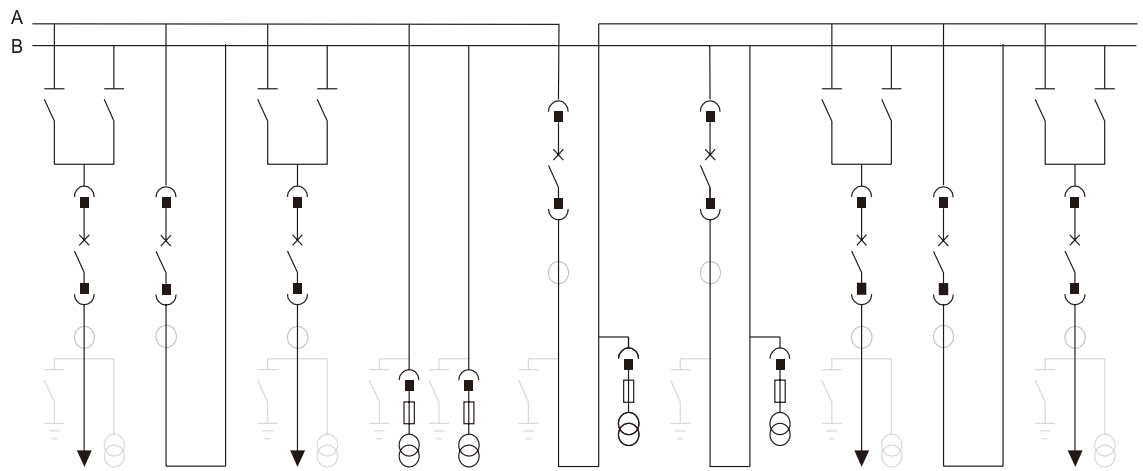
带母联母线分断系统
