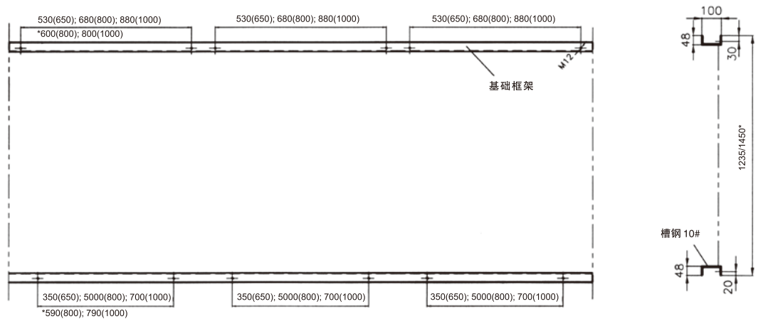
图17.4: 柜宽为1,000 mm, 800 mm, 650 mm三种柜型的基础框架典型加工图
