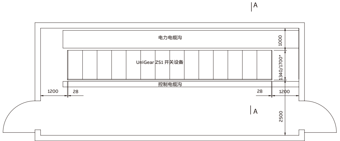
图17.1: 配电室典型平面布置图
