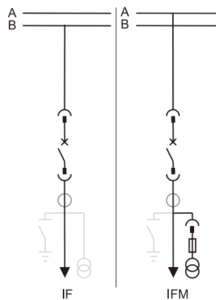
3 IF/IFM-母线B进线(复式)
