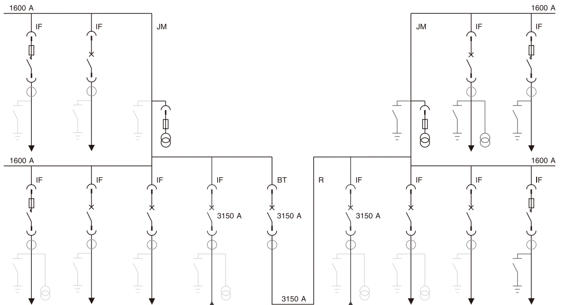
— 单、双层柜组合方案
